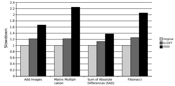
(d) Issue width 8
